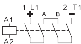
Schaltschema (4 Kontakte)
