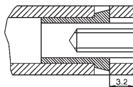
Schraube 4 Umdrehungen herausdrehen
