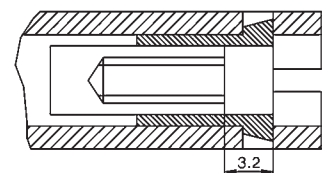
Schraube 4 Umdrehungen hineindrehen
