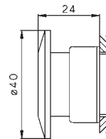
Pilz-Druck-Zug-Taster Ø40mm mit Schlüssel
